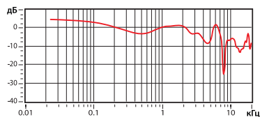
График АЧХ
