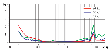
График КНИ
